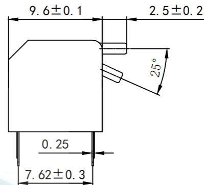
长拨柄(L)
