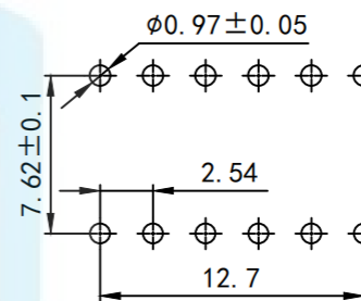
PCB开孔
