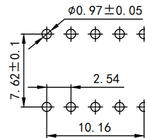
PCB开孔
