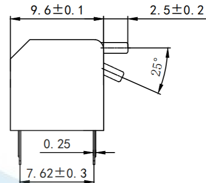
长拨柄(L)
