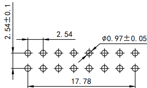
PCB开孔
