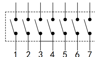
电路图
