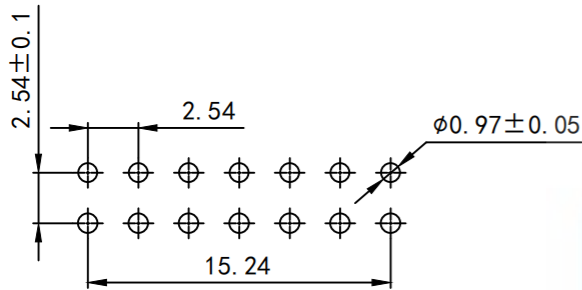
PCB开孔
