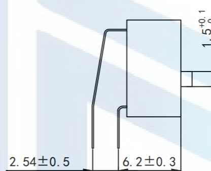
高推钮 (E)
