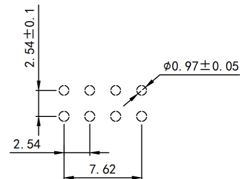
PCB开孔
