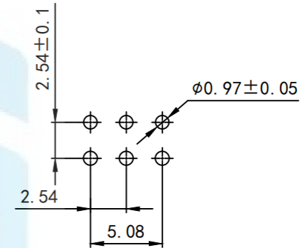
PCB开孔
