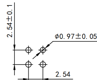
PCB开孔
