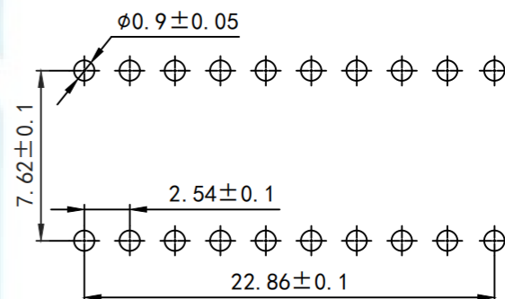
PCB开孔
