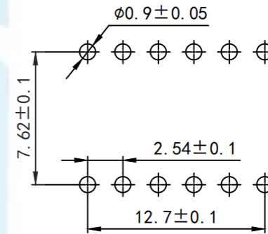
PCB开孔
