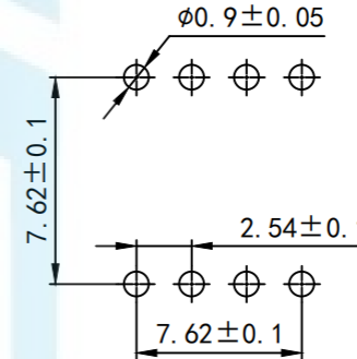
PCB开孔
