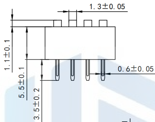
高推钮 (E)
