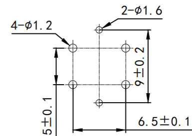
线路板安装孔尺寸
