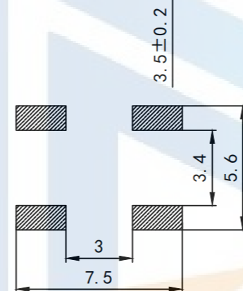
PCB. 焊接图
