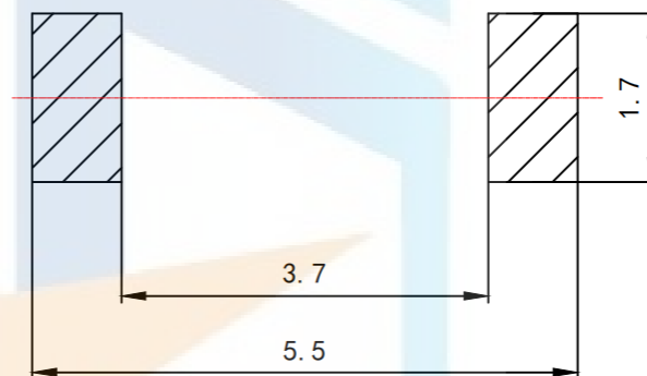
PCB. 焊接图
