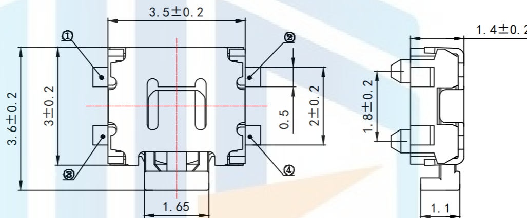
PCB. 焊接图
