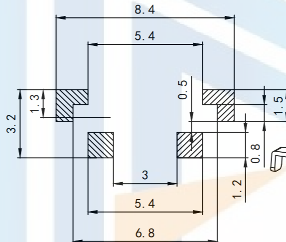
PCB. 焊接图
