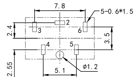
线路板开孔尺寸
