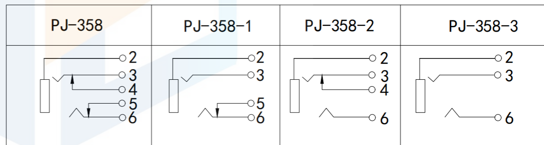
电路原理图
